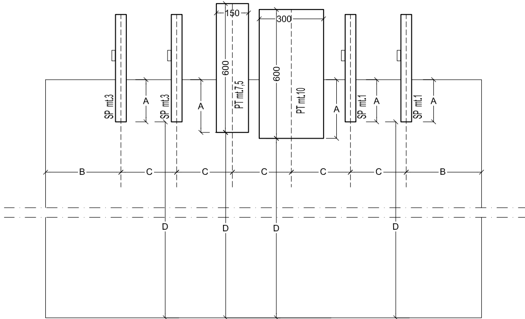
PLANIMETRIA
