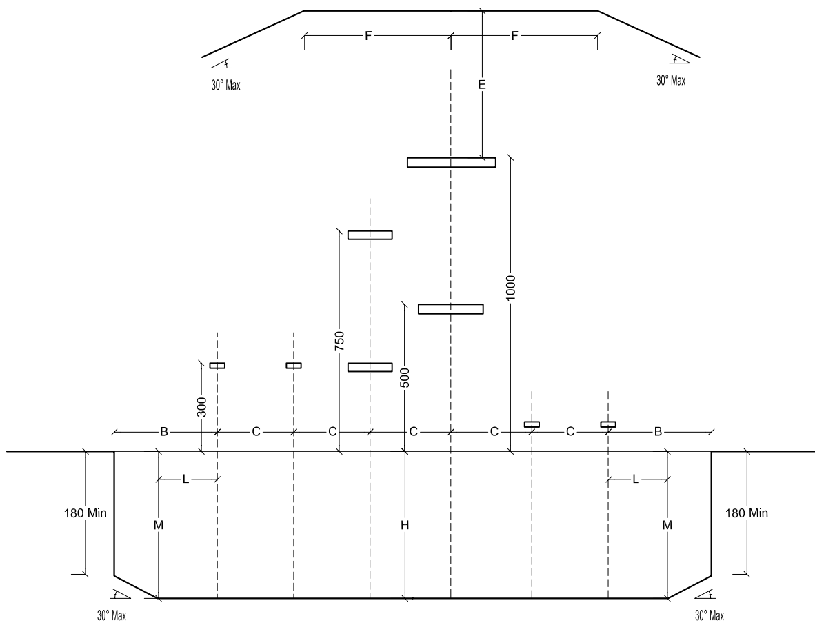
SEZIONE TRASVERSALE
